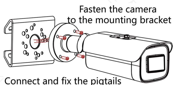
Figure 3-1 カメラの固定
