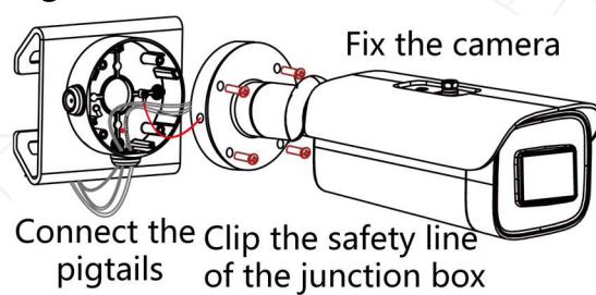
Figure 3-5 カメラの固定
