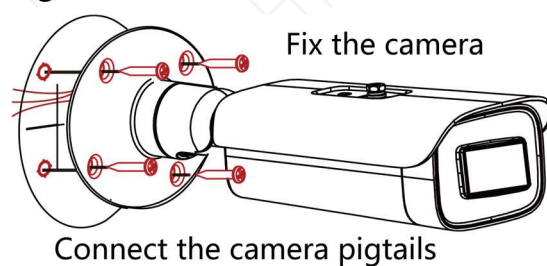
Figure 3-10 カメラの固定
