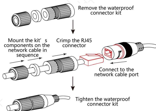
Figure 3-13 ネットワークケーブルの接続
