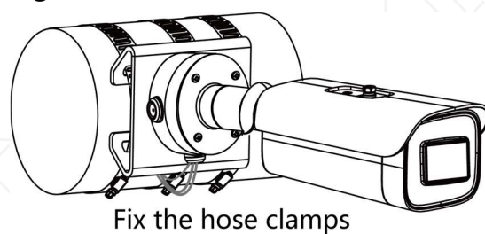
Figure 3-6 ホースクランプを固定します
