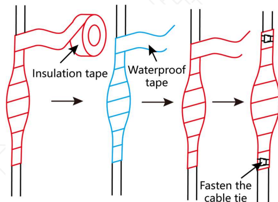
Figure 3-9 絶縁テープ・防水テープの巻き付け
