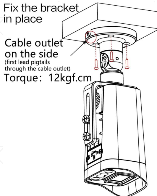
Figure 3-5 ブラケットの固定
