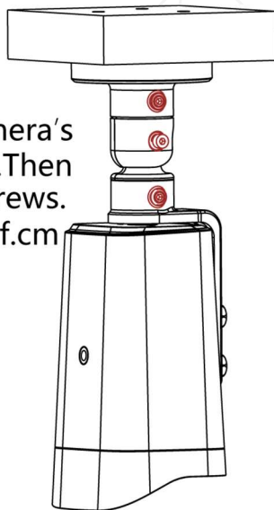
Figure 3-6 カメラの向きの調整
