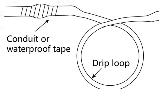
Figure 3-10 ドリップループ
