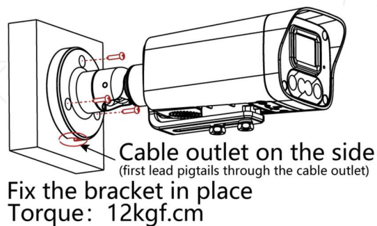
Figure 3-2 ブラケットの固定
